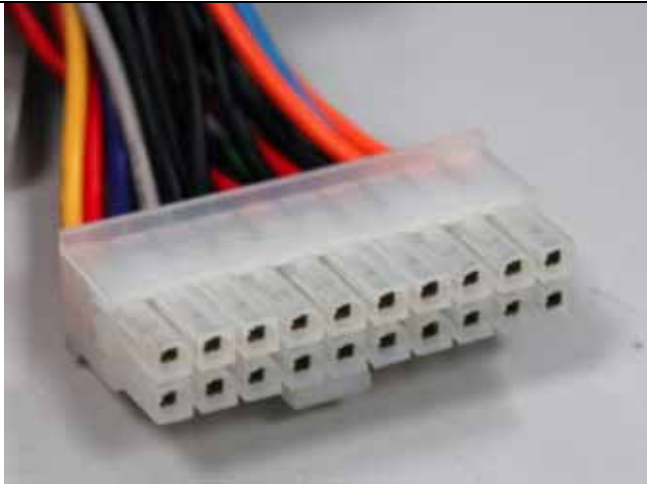
connettore 20 poli
