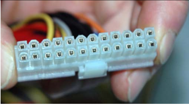
connettore 20+4
